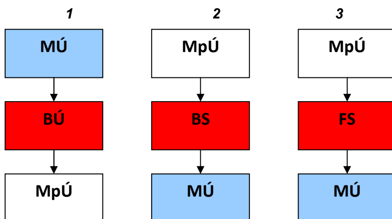
Obrázek 1: Schéma základních procesů MBÚ
